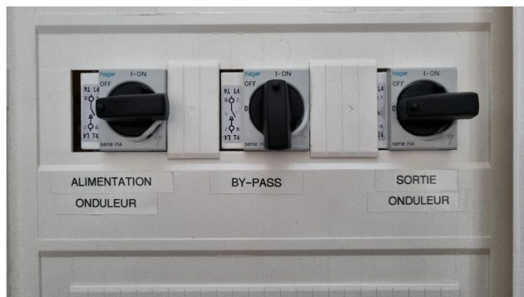
Figure 1 : fonctionnement en bypass externe
